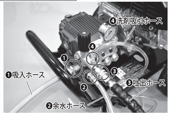
各ホースの取付全体図
