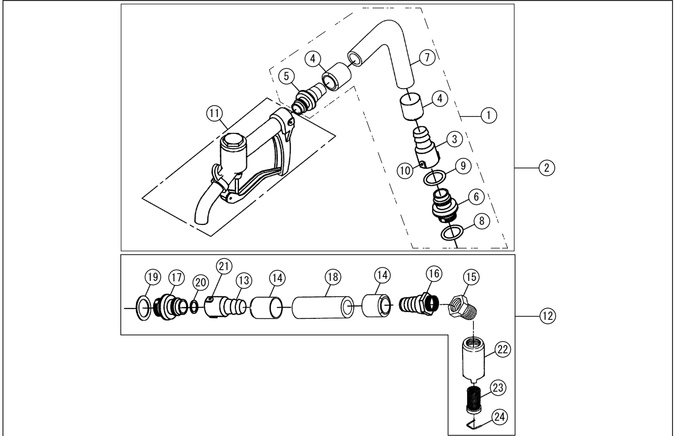
型式名 FS-20 T型ホースセット (014862303)
