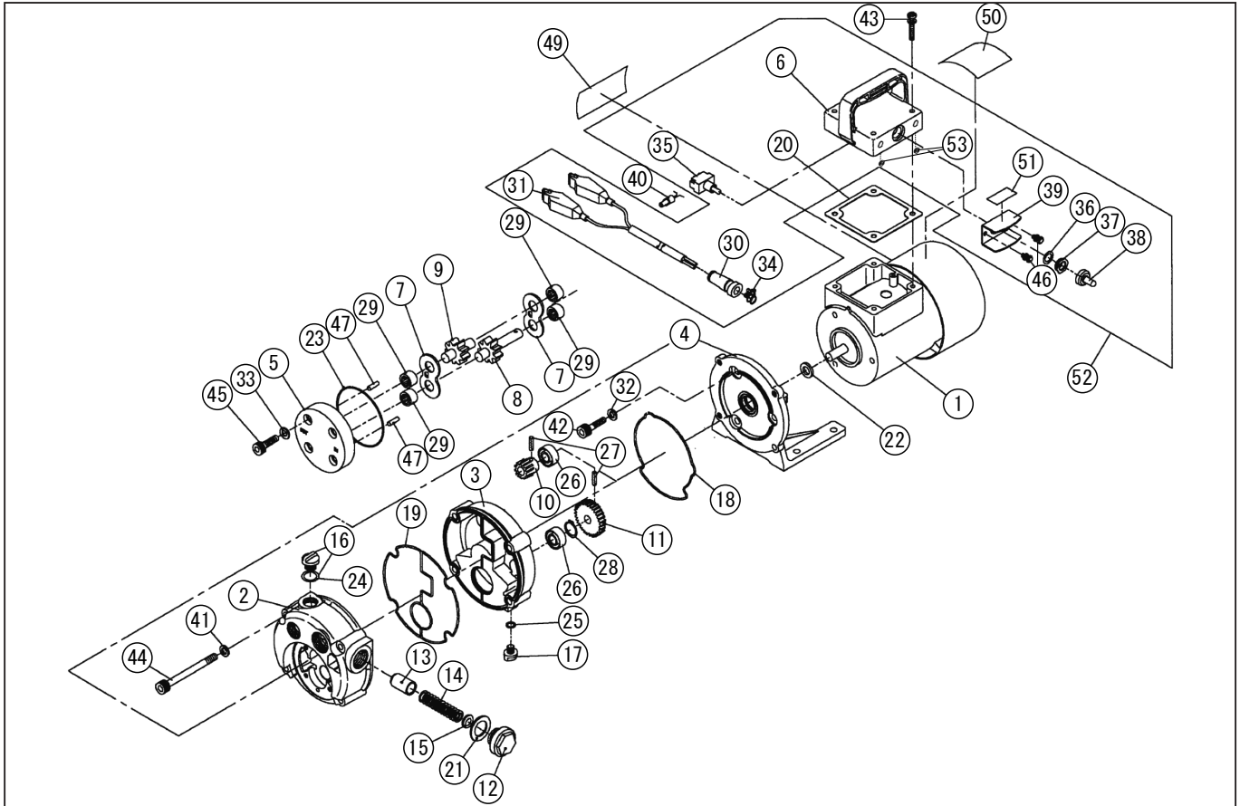
型式名 GM-2524H-AAA-5 (015852628)
