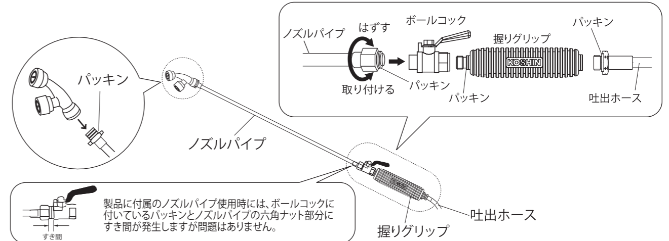
カバー付泡状除草噴口 (ES-10PDX/15PDX/20PDX) 泡状散布
