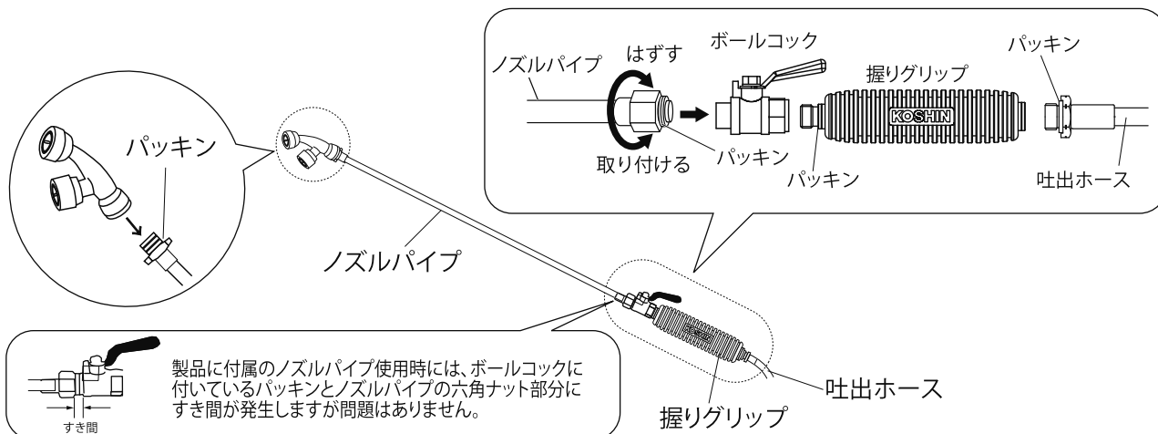
カバー付泡状除草噴口 (ES-10PDX/15PDX/20PDX)
