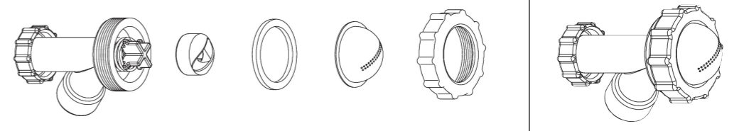
【シャワー噴口分解図】
