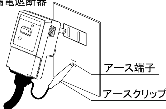
漏電遮断器
