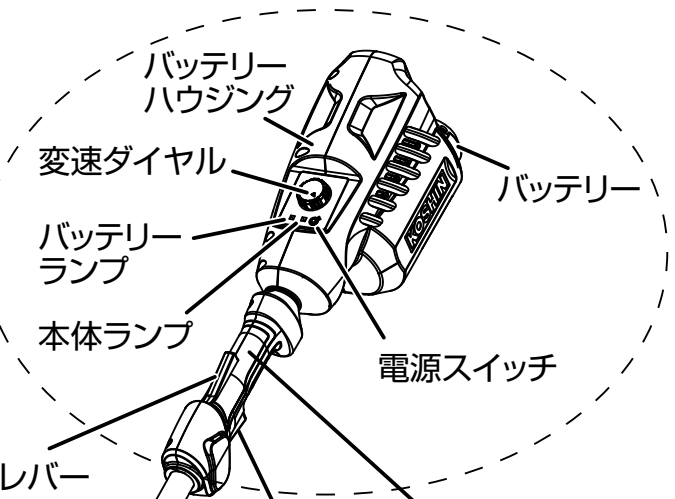
バッテリー取付け部 SBC-3650LBの場合
