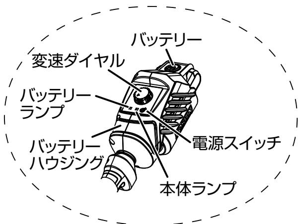
バッテリー取付け部 SBC-1825LBの場合
