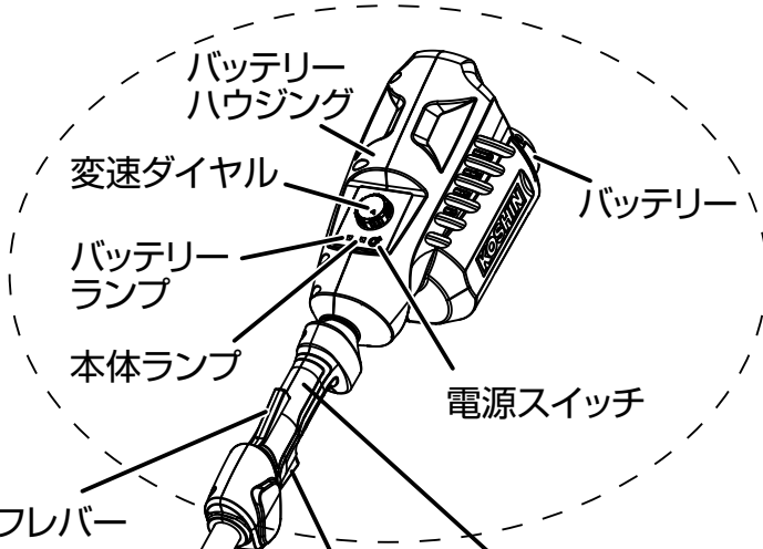
バッテリー取付け部 SBC-3650Lの場合
