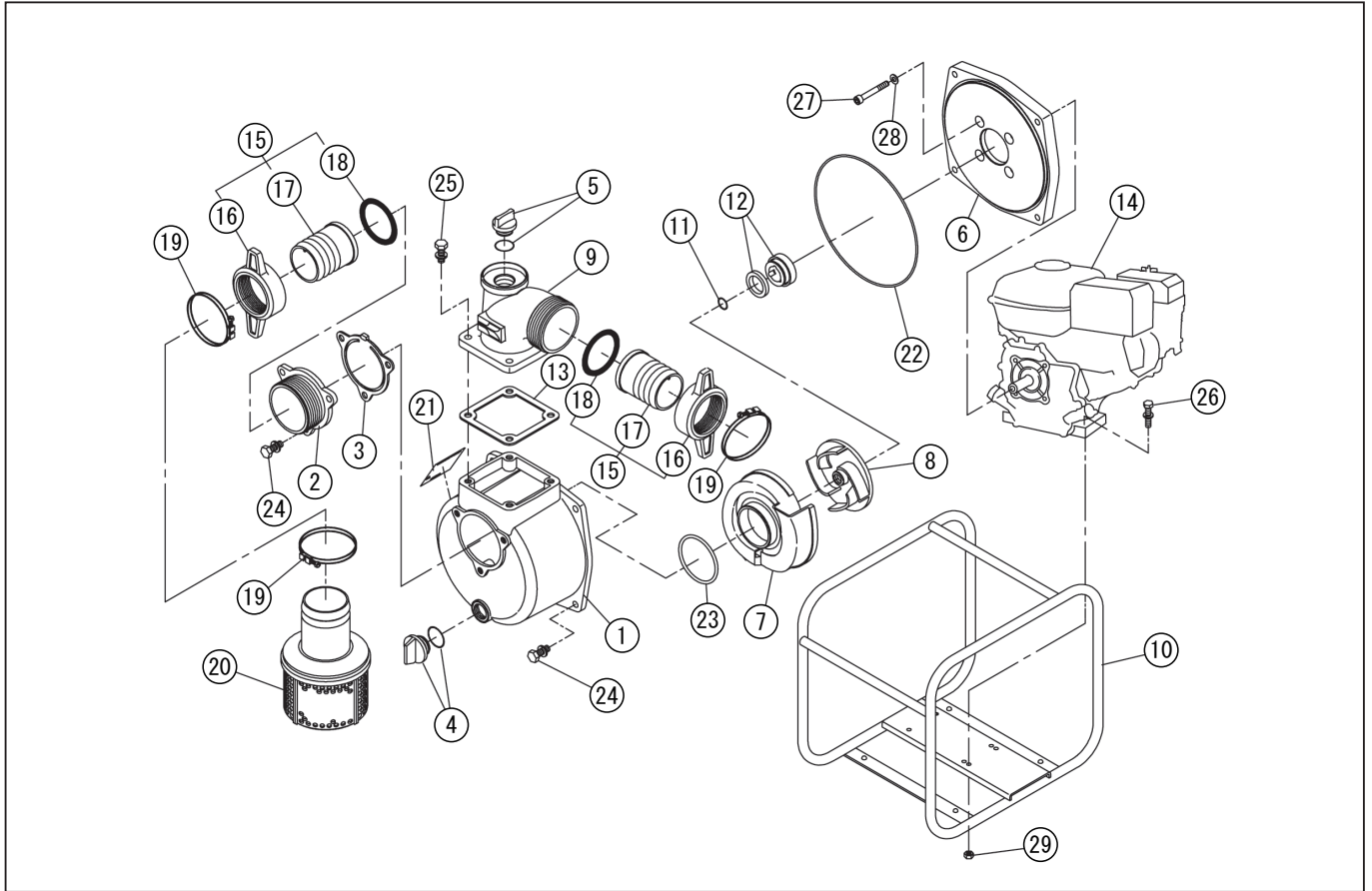
DWG No.066850410 MODEL : SEH-80X FORM : SEH-80X-BCE-2
