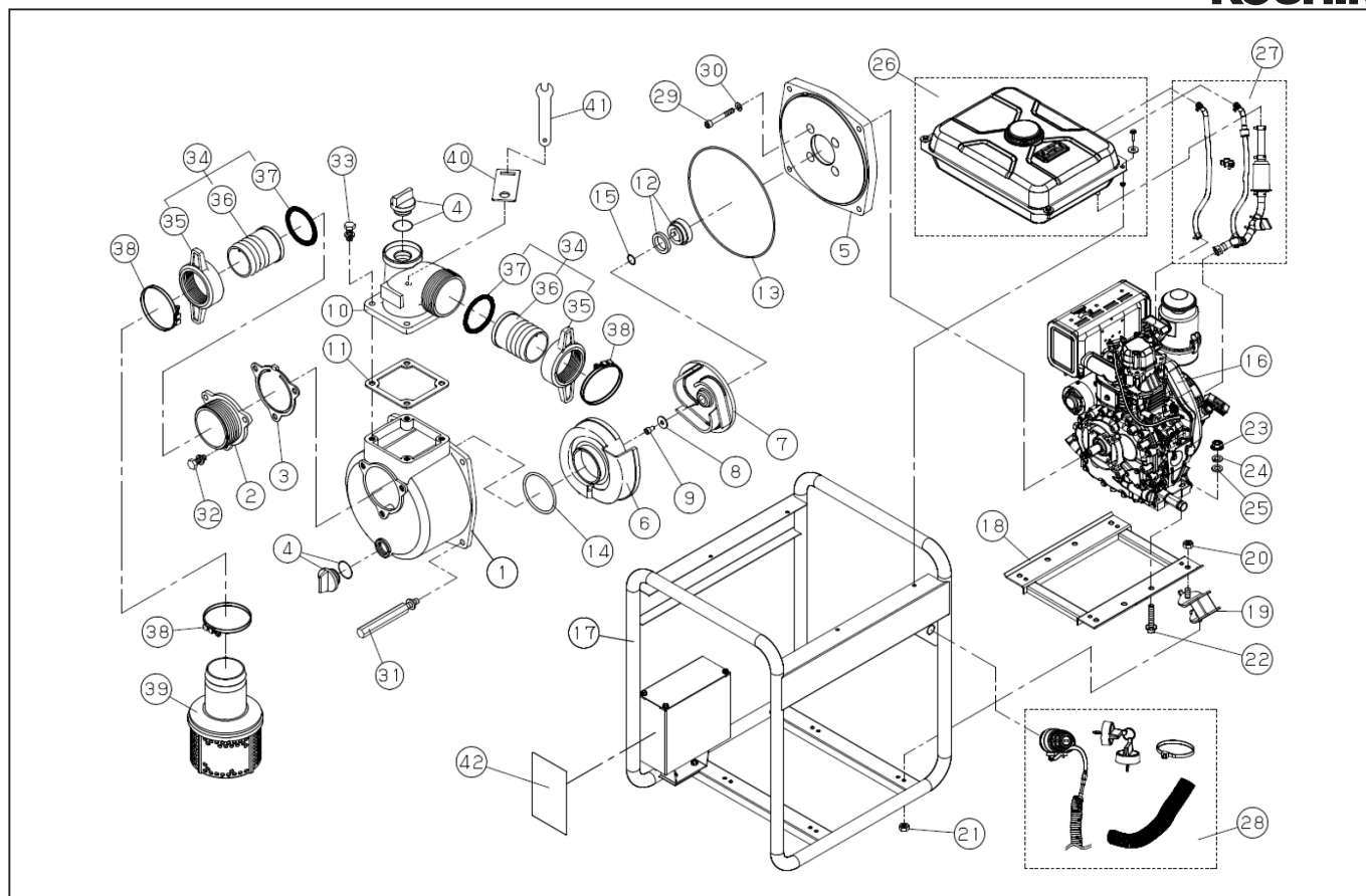
DWG No.013865101 MODELE : STV-50DS FORM : STV-50DS-BAA-0 (KD300)
