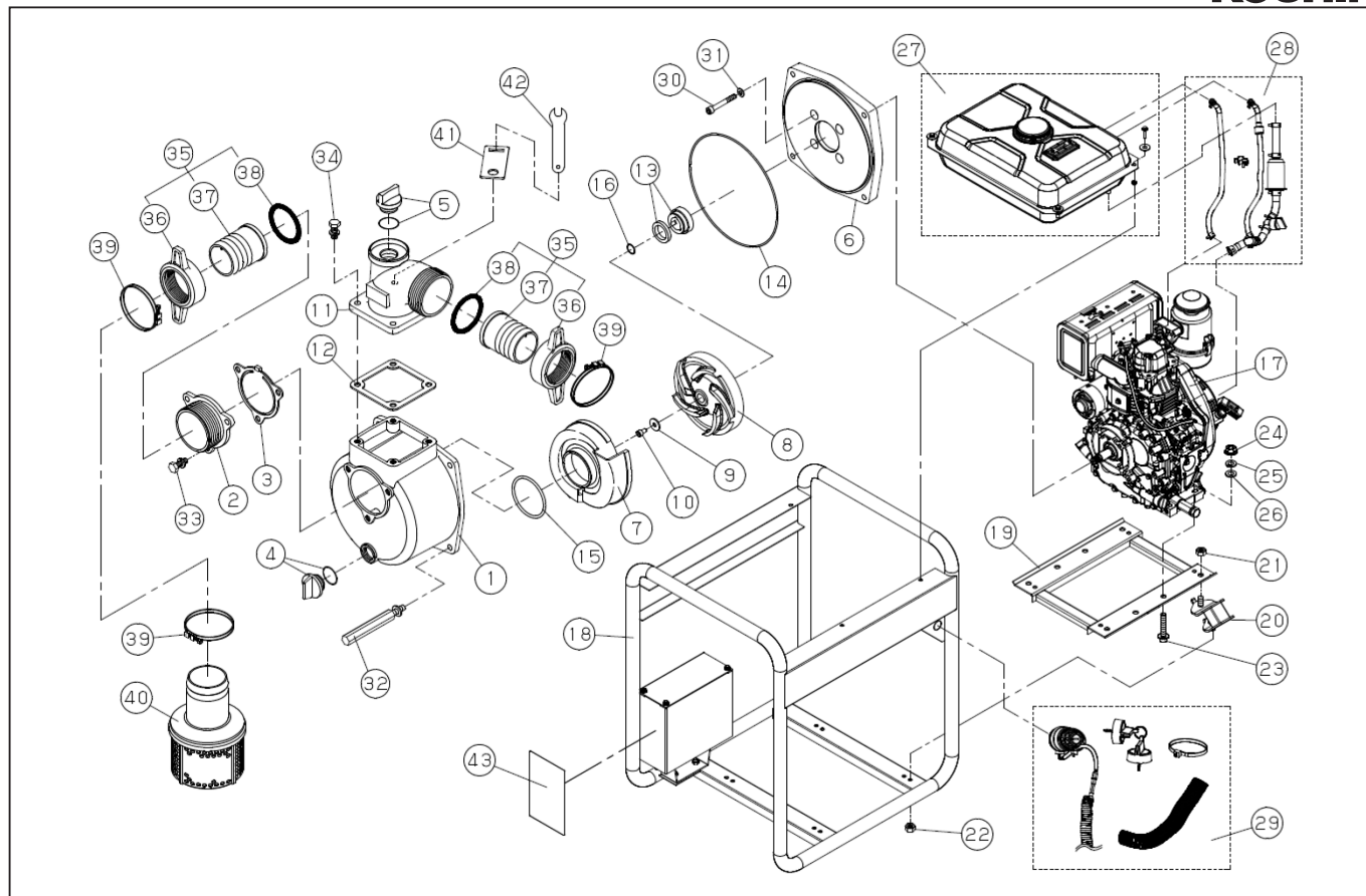
DWG No.013865201 MODELE:STV-80DS FORM:STV-80DS-BAA-0 (KD300)
