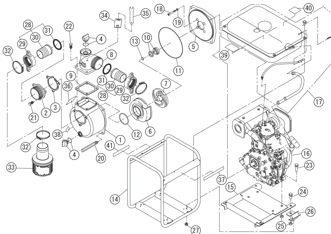
DWG No.012942901 MODELE:STY-50D FORM:STY-50D-BAB-0
