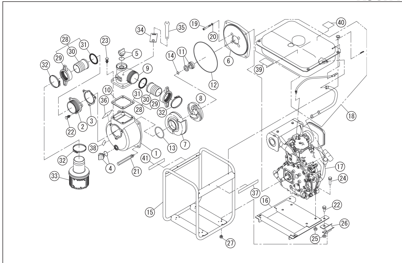
DWG No.012943004 MODELE:STY-80D FORM:STY-80D-BAB-1
