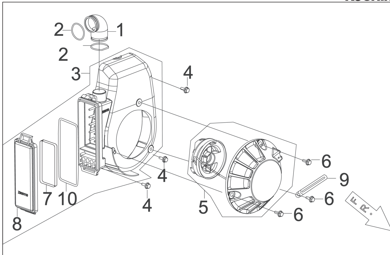
型式名 GV-9SE-AAA-0 (065864501) ファンカバー、リコイルスターター
